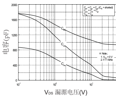
图5. 电容特性
