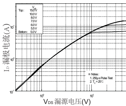
图1. 通态特性
