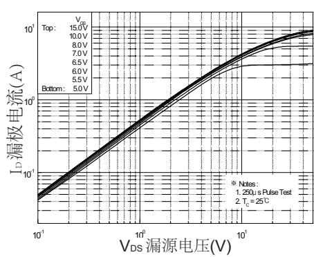
图1. 通态特性
