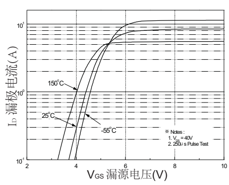
图2. 变化特性
