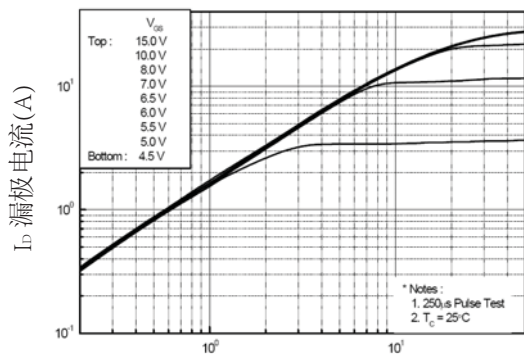
图1. 通态特性
