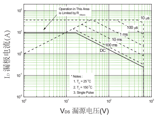
图9-1. 最大安全使用范围(TO-220)
