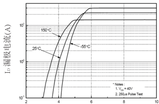
图2. 变化特性
